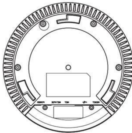
图 1 GWN7610/7600 端口
