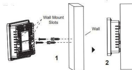
图 20 GWN7602 壁挂式
